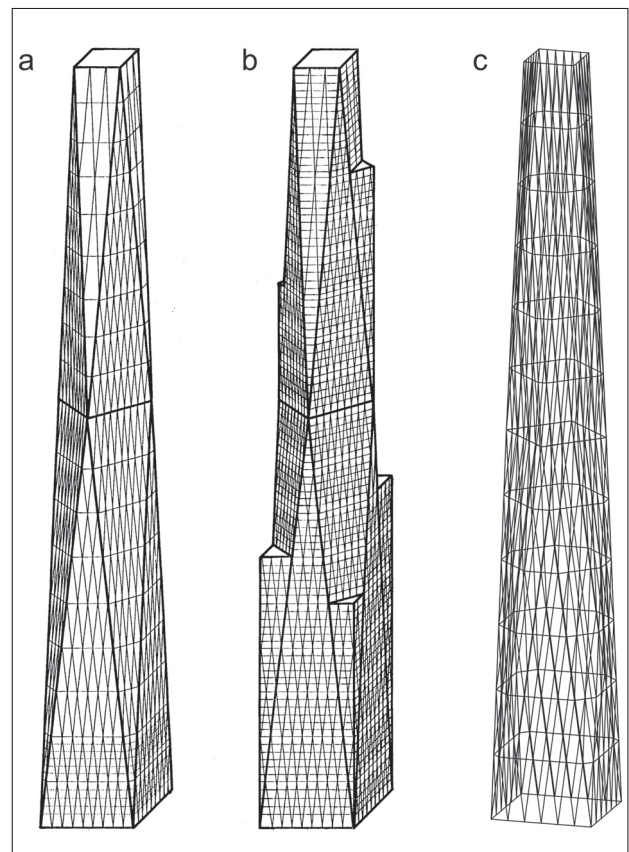
8. Propozycje bardziej złożonych postaci systemu wielościanu ramowego
