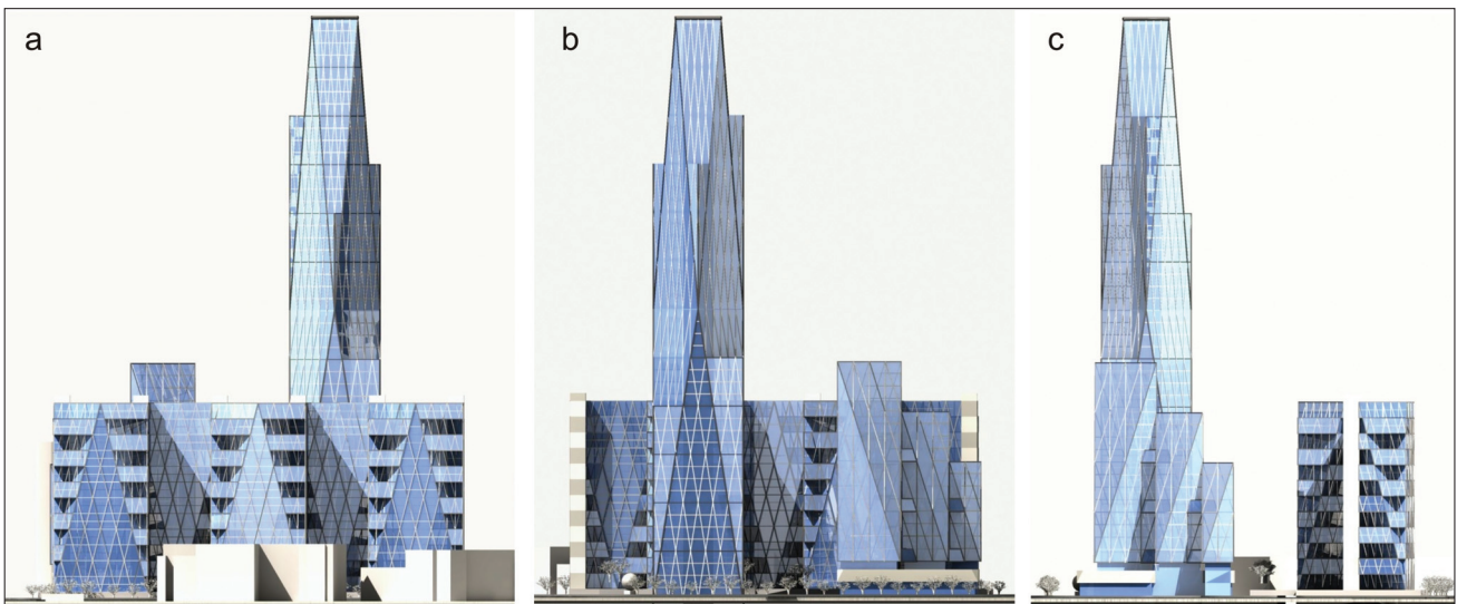
11. Elewacja: a. zachodnia; b. wschodnia; c. północna wielofunkcyjnego zespołu budynków 11. Elevations: a. west; b. east; c. north of the multifunctional complex of buildings
